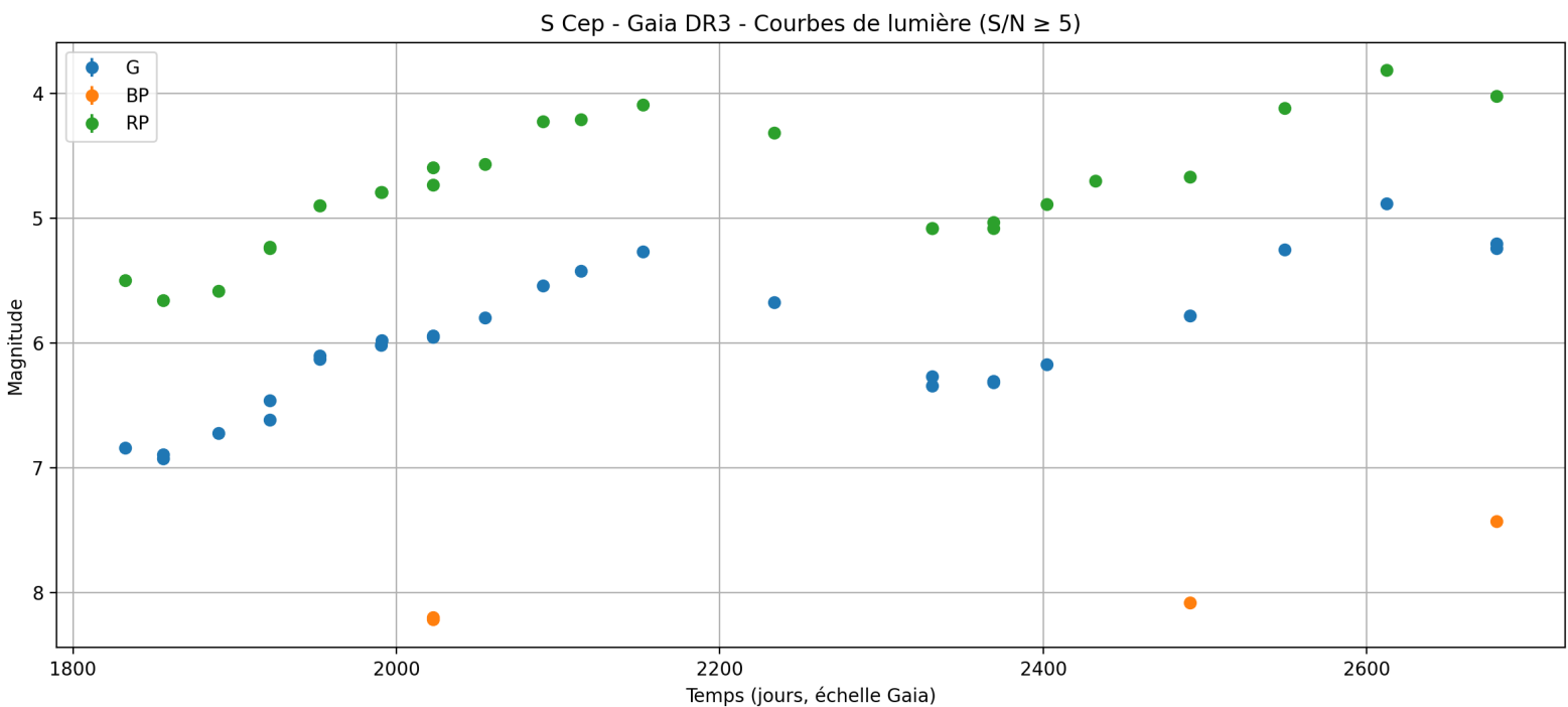
Figure 1 – Courbe de lumière Gaia pour S Cep
